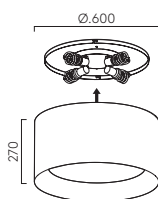
BEVEL ROUND 600
