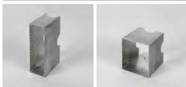
55 WALL BOX 6013001 H:165mm W:51mm D:100mm 90 WALL BOX 6013002 H:108mm W:87mm D:100mm
